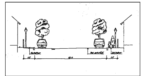
Sektion A-A.
