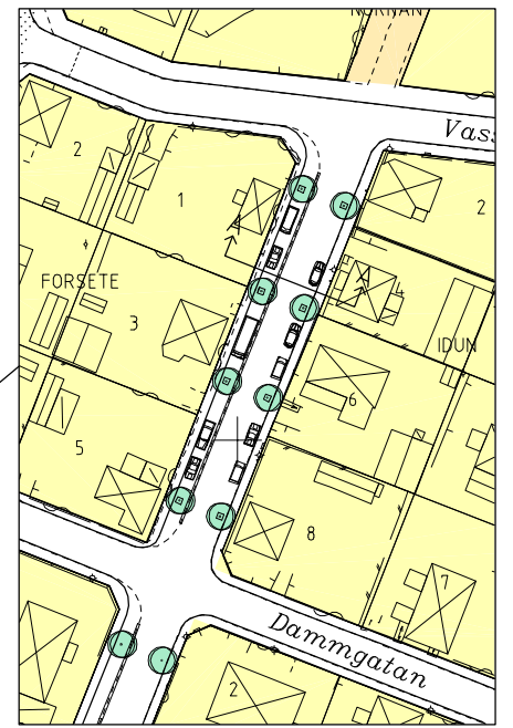
Förslag till utformning av del av Hjärtumsgatan Skala 1:500
