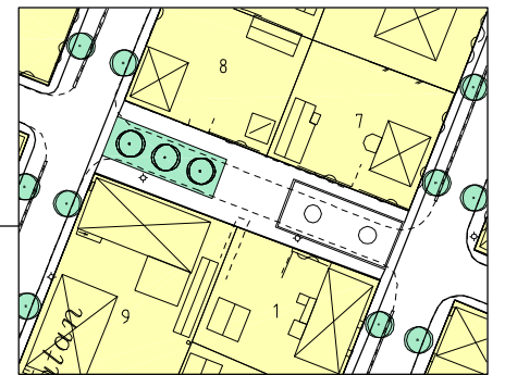
Förslag till utformning av del av Dammgatan. Skala 1:500.
