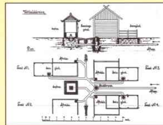
Plan och sektion genom sophus och slaskinrättning
